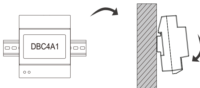
Montare pe sina DIN
