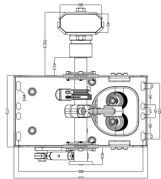
Dimensiuni mecanism
