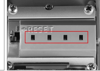
2 Rotiti cifrele urmarind ca pe spatetele capacului sa se alinieze 4 indicatoare rosii
